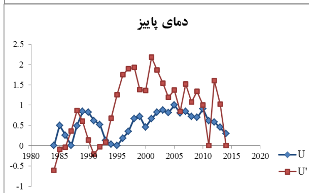
شکل ۳- نمودار من-کندال دمای فصلی و سالانه تهران طی دوره (۱۹۸۴-۲۰۱۴)
