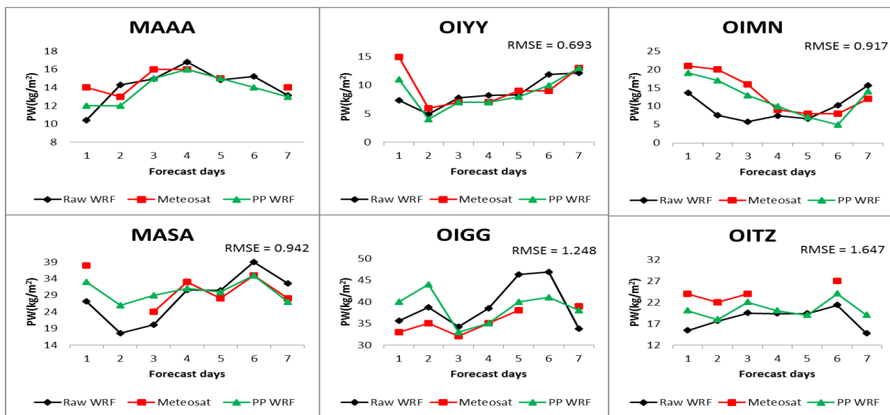
شکل ۳- مقایسه فراسنج آب قابل بارش پس پردازش شده (خط سبز)، خام (خط مشکی) و ماهواره Meteosat (خط قرمز) طی ۷ روز پیش‌بینی در شهرستان‌های: (a) اراک، (b) یزد، (c) بجنورد، (d) ساری، (e) رشت و (f) زنجان
