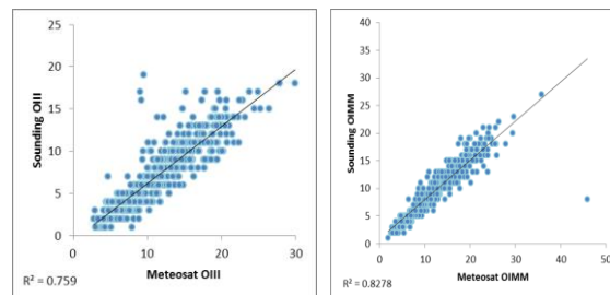
شکل ۱- مقایسه فراسنج آب قابل بارش ماهواره METEOSAT و رادیوسوند تهران
