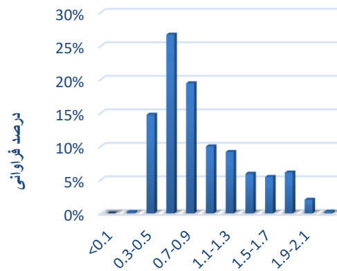
ارتفاع موج بر حسب متر
