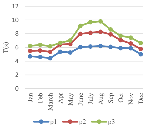
شکل ۵: میانگین ماهانه پریرود موج بر حسب ثانیه (در دوره آماری ۲۰۱۳-۲۰۱۵ و ۲۰۱۹-۲۰۲۱) در هر سه نقطه
