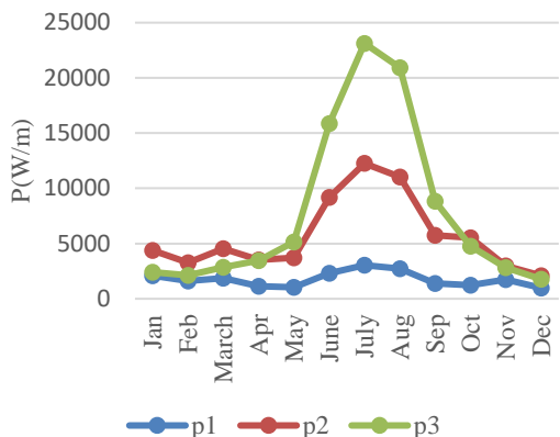
شکل ۶- میانگین ماهانه توان موج بر حسب وات بر متر (در دوره آماری ۲۰۱۳-۲۰۱۵ و ۲۰۱۹-۲۰۲۱) در هر سه نقطه
