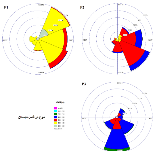
شکل ۱۰: گلموج سه نقطه مورد مطالعه در فصل تابستان
