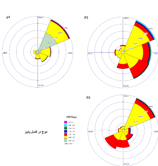
شکل ۱۲: گلموج سه نقطه مورد مطالعه در فصل پاییز
