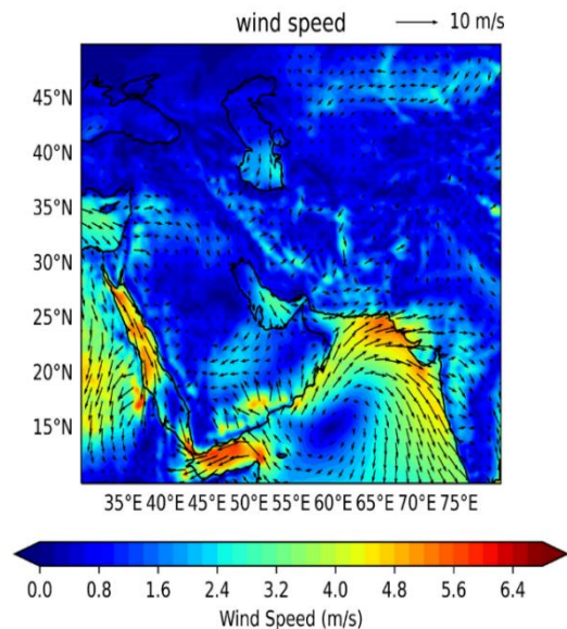
شکل ۷: میانگین جهت و اندازه سرعت بر حسب متر بر ثانیه در فصل بهار (از مارس تا می در دوره آماری ۲۰۰۵-۲۰۱۵)
