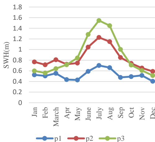
شکل ۴- میانگین ماهانه ارتفاع موج شاخص بر حسب متر (در دوره آماری ۲۰۱۳-۲۰۱۵ و ۲۰۱۹-۲۰۲۲) در هر سه نقطه
