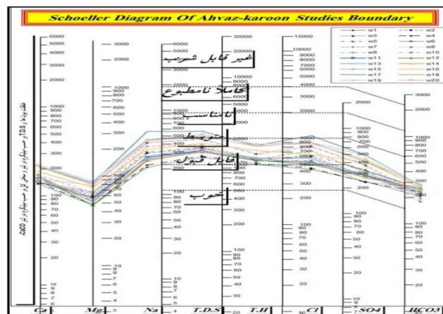
شکل ۲- نمودار شولر رودخانه کارون از سال ۷۲ تا ۹۲
