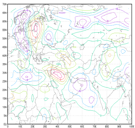
الف- تراز ۵۰۰ هکتوپاسکال
