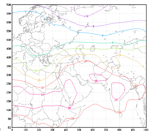
ج- تراز ۸۵۰ هکتوپاسکال
