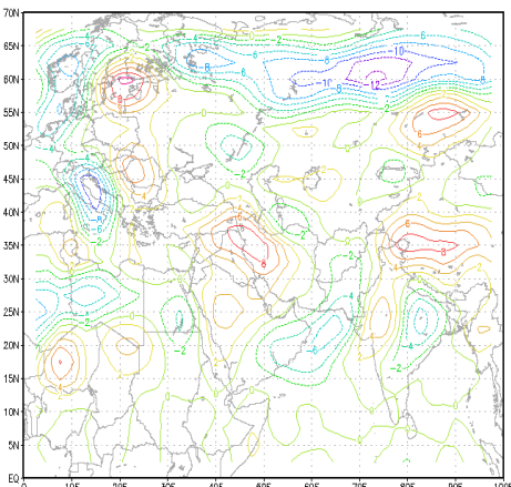
ب- تراز ۷۰۰ هکتوپاسکال
