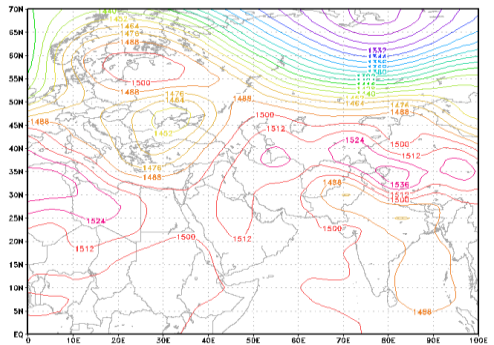
ج- تراز ۸۵۰ هکتوپاسکال
