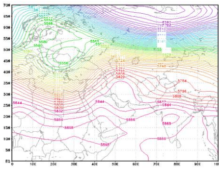
الف- تراز ۵۰۰ هکتوپاسکال
