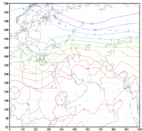
ب- تراز ۷۰۰ هکتوپاسکال
