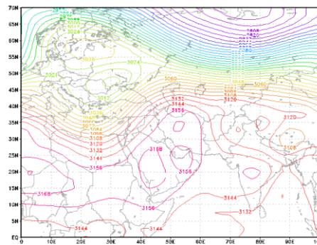
ب- تراز ۷۰۰ هکتوپاسکال
