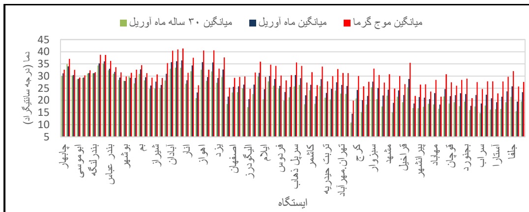
شکل (۲): سری میانگین دمای آوریل بلندمدت ۳۰ ساله، آوریل ۲۰۰۸ و میانگین دمای موج گرما ۲۲ تا ۳۰ آوریل ۲۰۰۸
