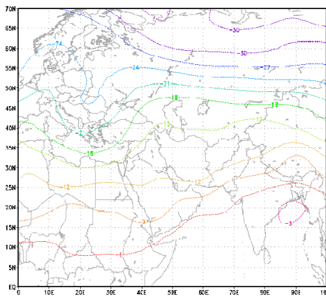
الف- تراز ۵۰۰ هکتوپاسکال
