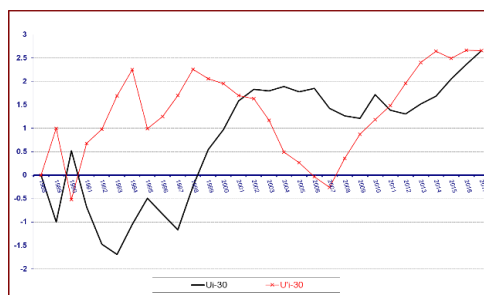
شکل ۷. تحلیل روند میانگین ایستگاهی دمای ایران
