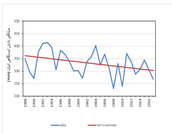
شکل ۴: برازش نمودار خط سن بر سری زمانی داده های میانگین بارش ایستگاهی ایران ۱۹۸۸-۲۰۱۷ میلادی
