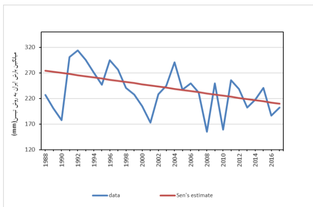
شکل ۵. تحلیل روند میانگین بارش ایران به روش تیسس ۱۹۸۸-۲۰۱۷ میلادی شکل ۶:- برازش نمودار خط سن بر سری زمانی داده های میانگین بارش تیسس ایران ۱۹۸۸-۲۰۱۷
