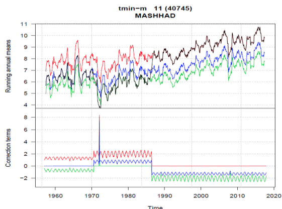
شکل ۱- سری اصلی (رنگ سیاه) و سری‌های اصلاح شده (نمودار بالا)، اصلاحات اعمال شده (نمودار پایین) برای پارامتر دمای می نیمم ایستگاه مشهد
