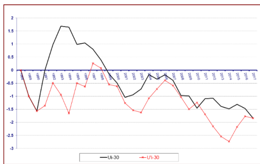
شکل ۳- تحلیل روند میانگین بارش ایستگاهی ایران
