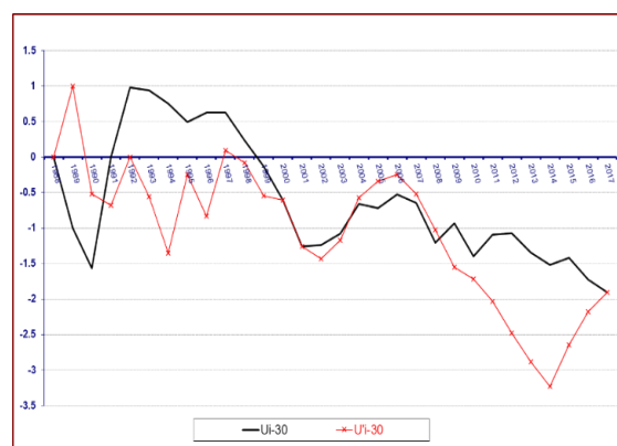
شکل ۵. تحلیل روند میانگین بارش ایران به روش تیسس ۱۹۸۸-۲۰۱۷ میلادی شکل ۶:- برازش نمودار خط سن بر سری زمانی داده های میانگین بارش تیسس ایران ۱۹۸۸-۲۰۱۷
