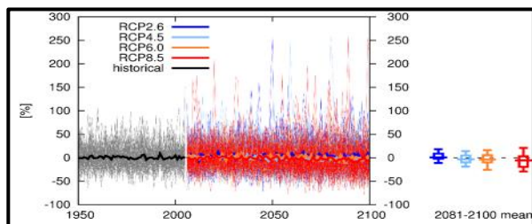
شکل ۱- تغییرات میانگین سالانه بارش ایران (%) تا سال ۲۱۰۰ نسبت به
