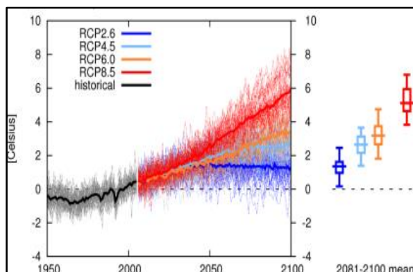
شکل ۲- تغییرات میانگین سالانه دمای ایران (oC) تا سال ۲۱۰۰ نسبت به دوره ۱۹۸۶-۲۰۰۵ تحت سناریوهای واداشت تابشی RCP.
