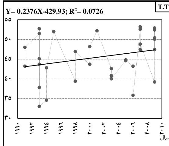
شکل ۴- نمودار پراکندگی شاخص‌های ناپایداری نسبت به سال‌های وقوعشان، در غرب کشور (۱۹۶۱-۲۰۱۰)
