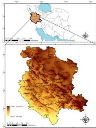
شکل ۱- موقعیت جغرافیایی منطقه و ایستگاه‌های هواشناسی مورد مطالعه در پژوهش شکل ۲- نمودار درخت خوشه‌بندی روزهای بارش فرین
