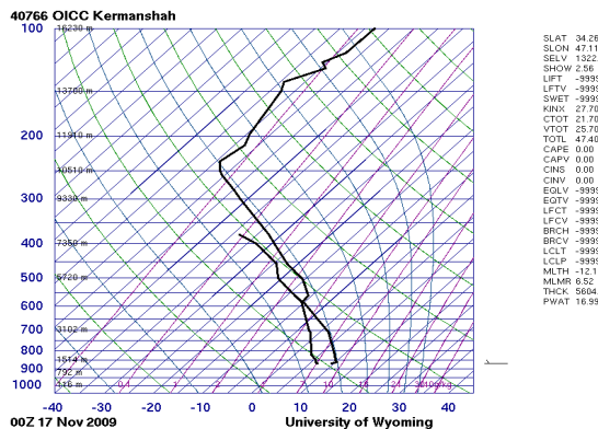
شکل ۳- نمودار اسکیتیوی مربوط به روز وقوع بارش سنگین در ایستگاه کرمانشاه (۱۷ نوامبر ۲۰۰۹)
