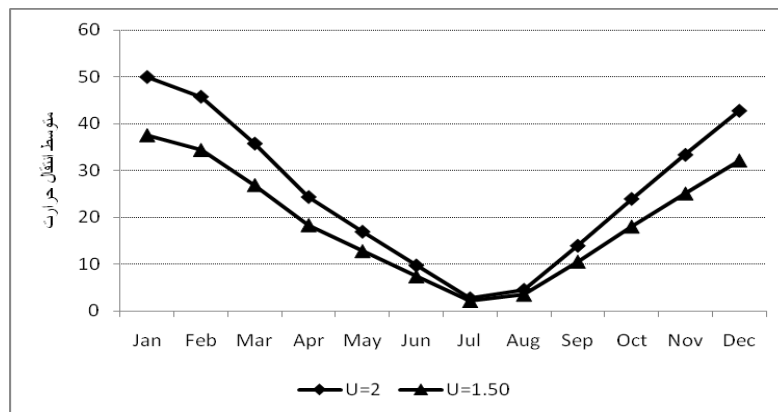
شکل ۸- متوسط انتقال حرارت از یک متر مربع بام با مصالح متفاوت در ماه‌های مختلف سال
