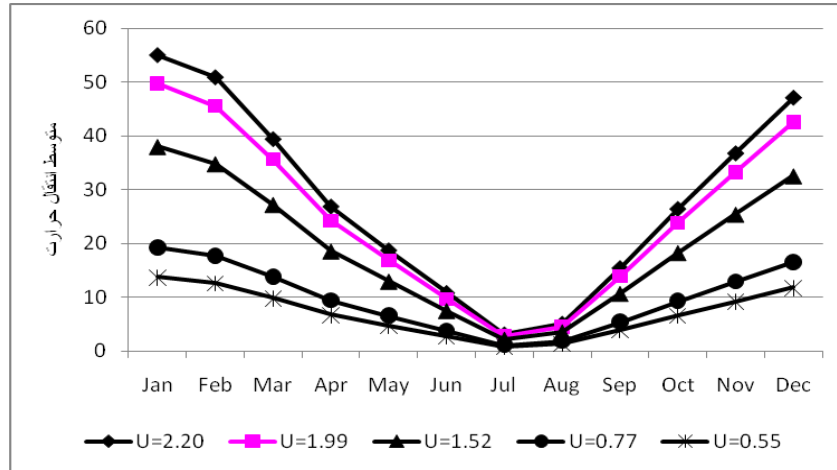
شکل ۷- متوسط انتقال حرارت از یک متر مربع دیوار با مصالح متفاوت در ماه‌های مختلف سال
