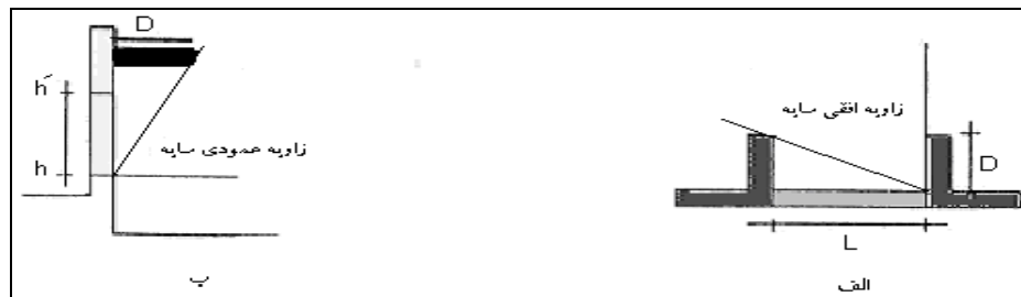
شکل ۲- محاسبه عمق سایه بان‌ها
