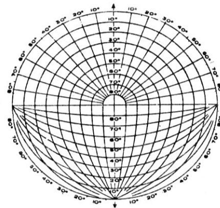
شکل ۵- انطباق مواقع گرم سال بر نمودار مسیر خورشید
