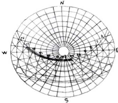
شکل ۶- نقاله سایه یاب
