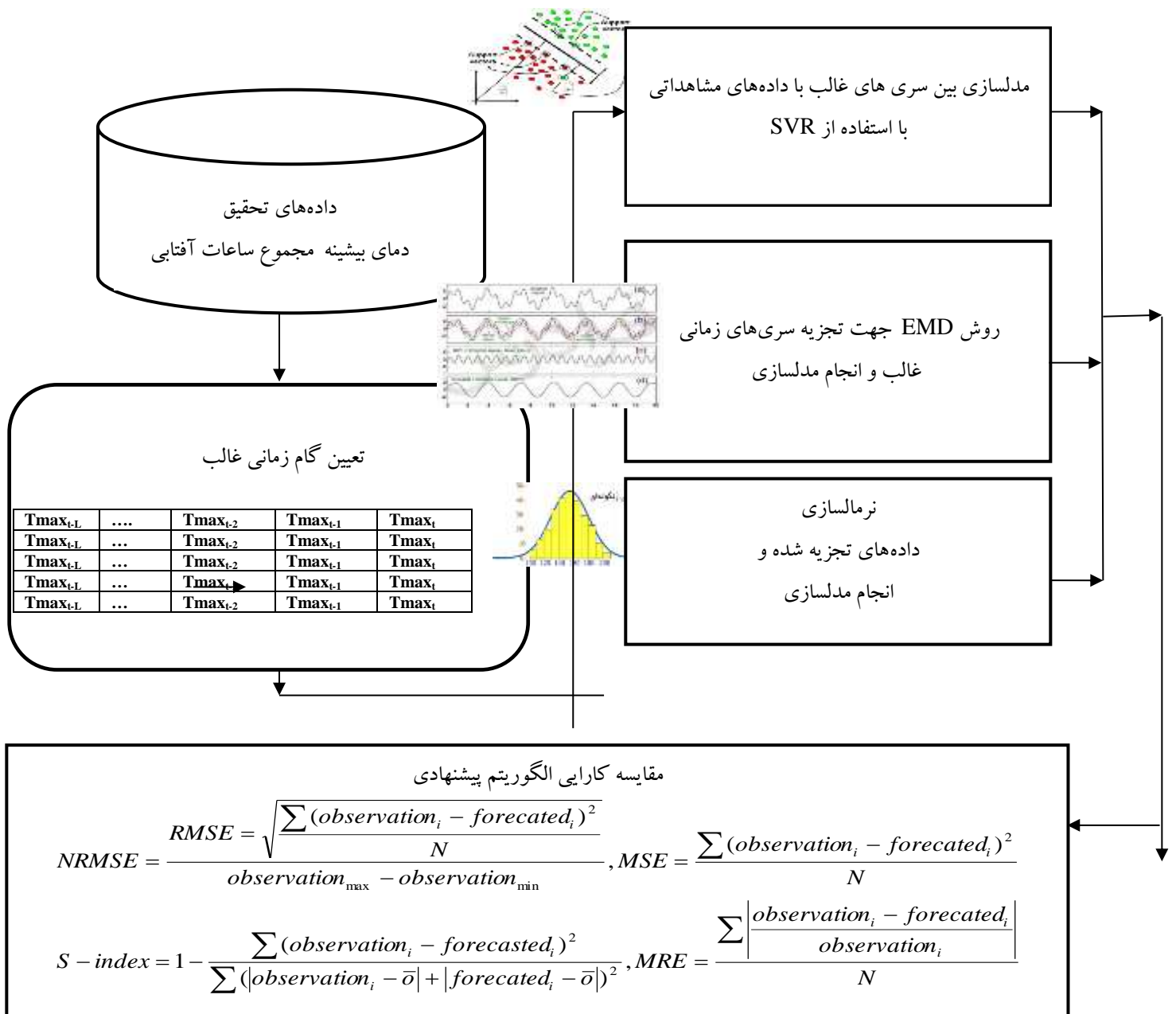
شکل ۲. روندنمای انجام تحقیق
