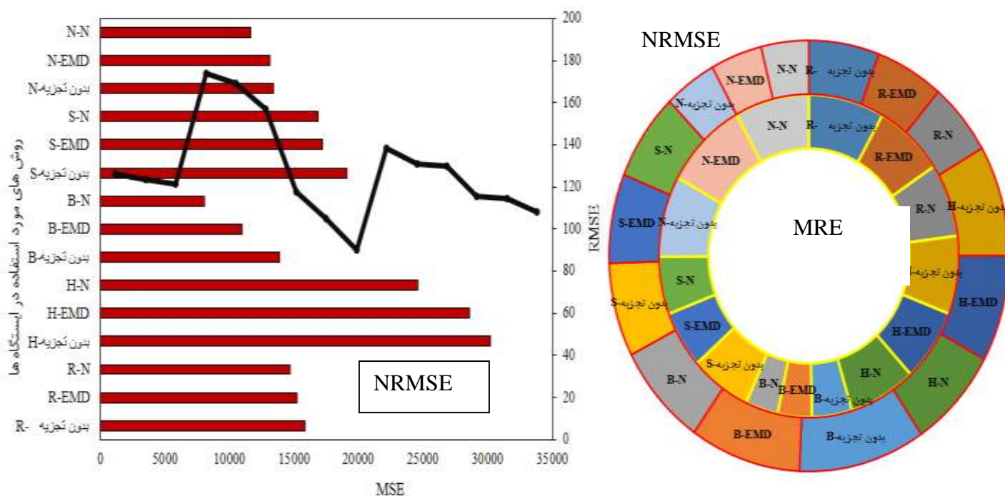
شکل ۸. بررسی تاثیر نرمال کردن سری های تجزیه شده ساعات آفتابی با آماره های ارزیابی در ایستگاه های مختلف
