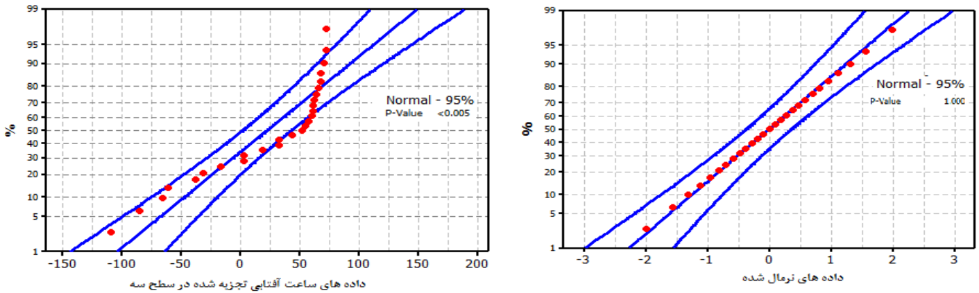
شکل ۶: نمودار احتمالاتی داده‌های تجزیه شده ساعت آفتابی سری اول، سطح تجزیه سه و داده‌های نرمال شده در ایستگاه رامسر
