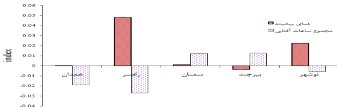
شکل ۹. مقادیر شاخص جهت تعیین بیش و کم برآورد الگوریتم پیشنهادی برای تمام داده‌ها و ایستگاه‌ها
