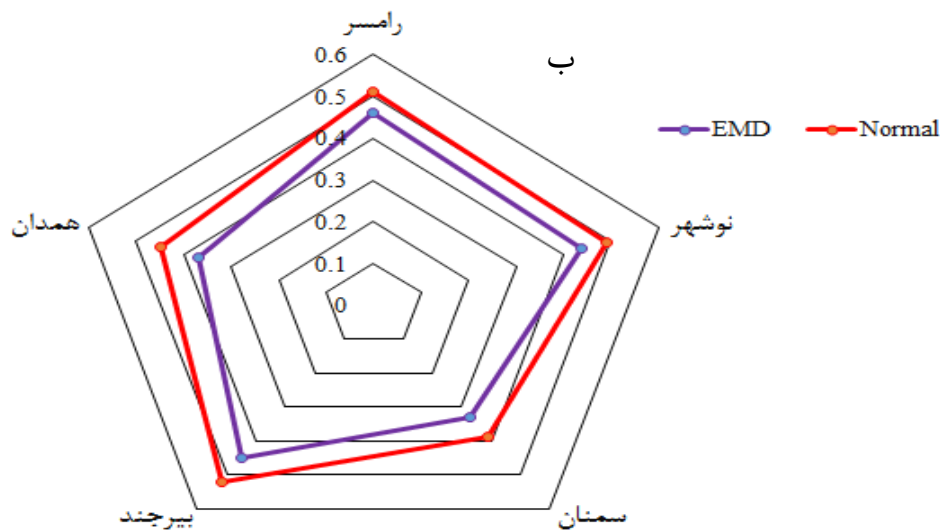
شکل ۷. آماره‌های ارزیابی سه روش مورد استفاده، بدون تجزیه، تجزیه با EMD و نرمال‌سازی در تمام ایستگاه‌ها (الف)، مقایسه مقدار S در بررسی عملکرد دو روش EMD و نرمال‌سازی (R: نماد رامسر، H: همدان، B: بیرجند، N: نوشهر، S: سمنان)
