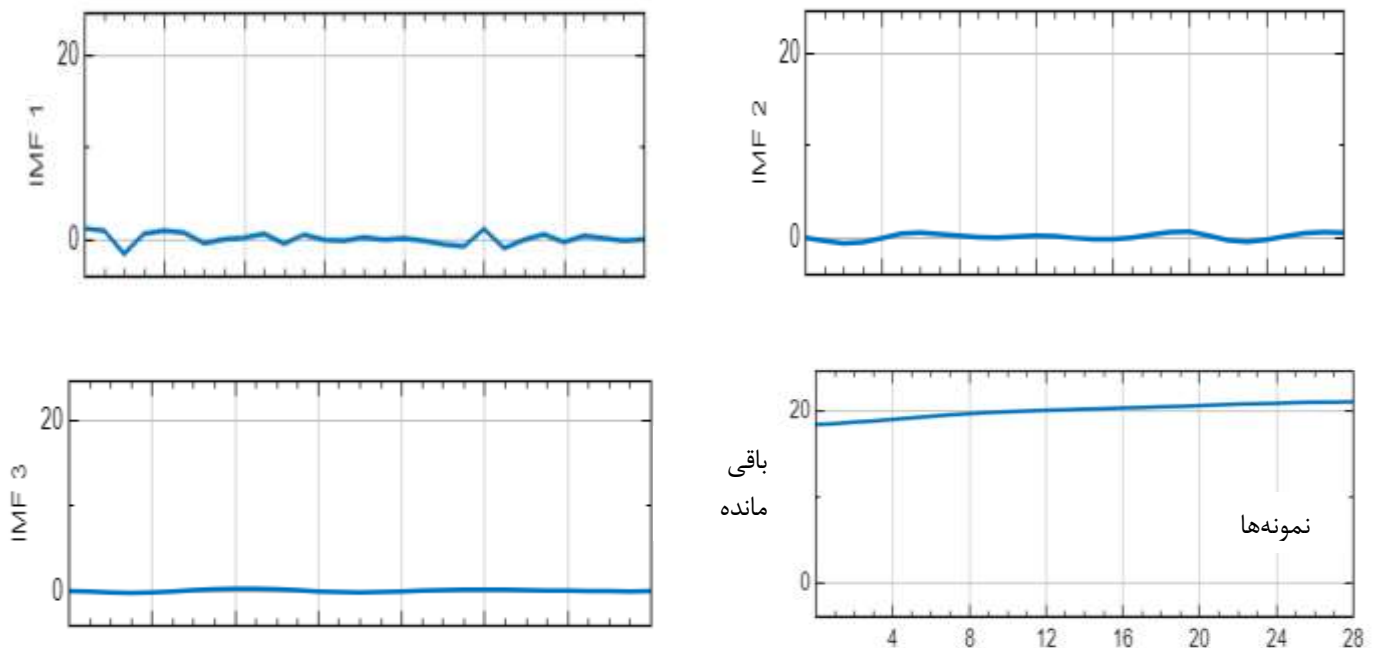
شکل ۵. زیر سری‌های حاصل از EMD برای دمای بیشینه در همدان برای تاخیر زمانی ۵
