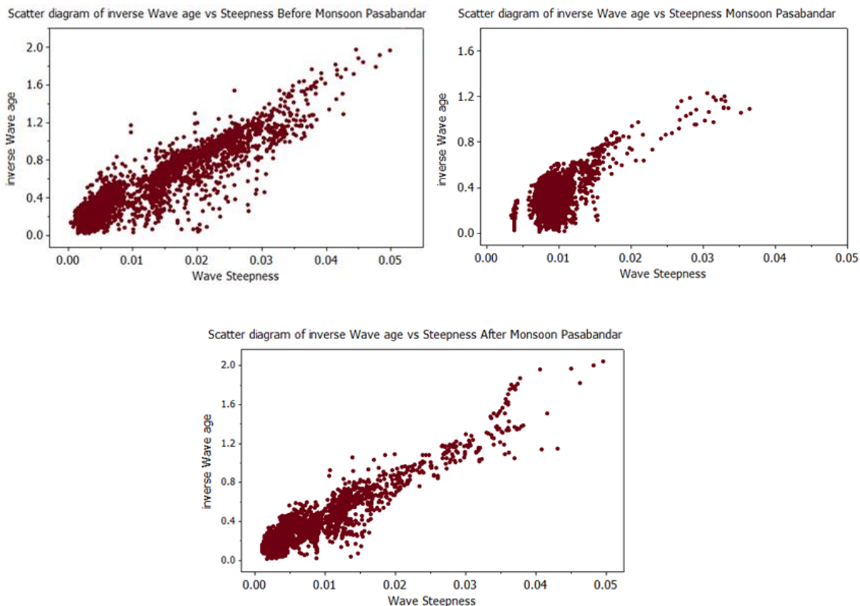
شکل ۱۶: توزیع توأم عکس سن موج - تیزی موج در فصول مختلف ایستگاه پسابندر
