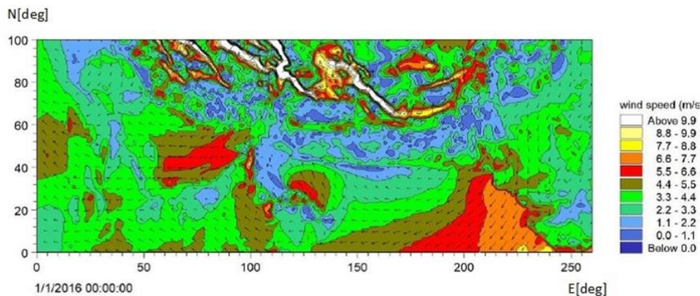
شکل ۳. میدان باد سال ۲۰۱۶ در سواحل مکران
