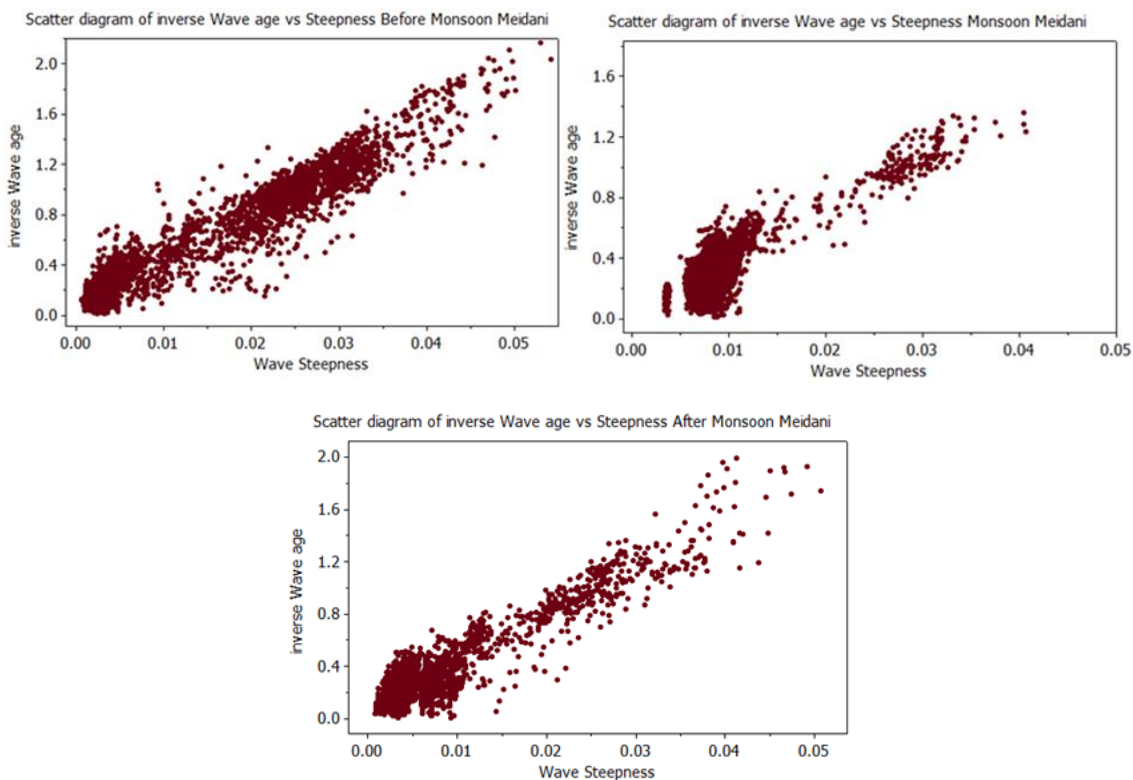
شکل ۱۷. توزیع توأم عکس سن موج - تیزی موج در فصول مختلف ایستگاه میدانی
