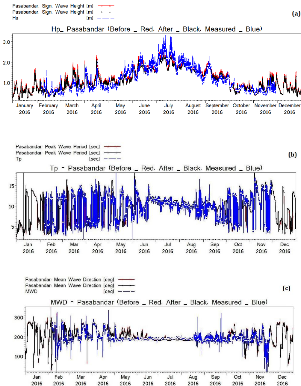
شکل ۴: مقایسه بین (a) ارتفاع موج شاخص H_s و (b) پریود پیک T_p و (c) جهت متوسط موج MWD ، اندازه گیری شده و شبیه سازی شده بعد از کالیبراسیون با ضرایب سفیدک موج تحت عنوان WC_4
