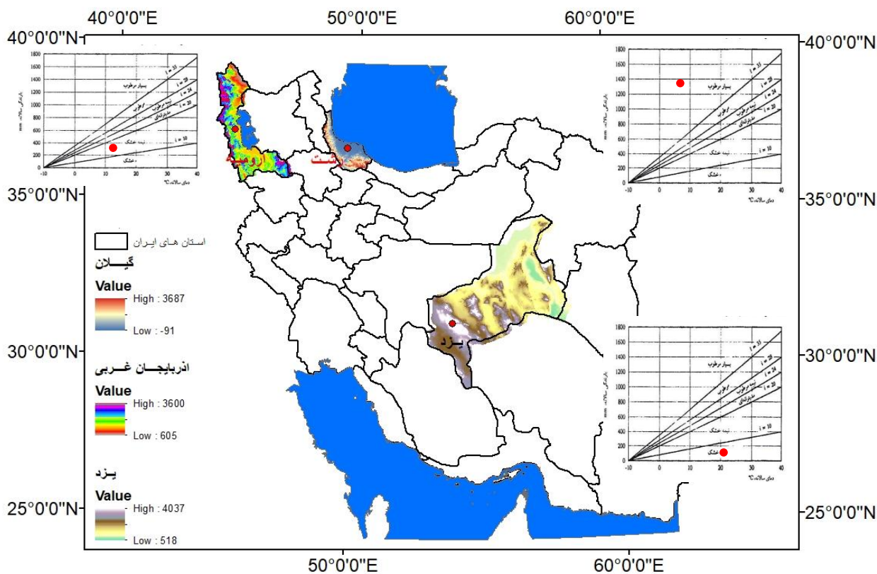
شکل ۱: موقعیت ایستگاههای مطالعاتی در کشور و اقلیم نمای دومارتن ایستگاهها
