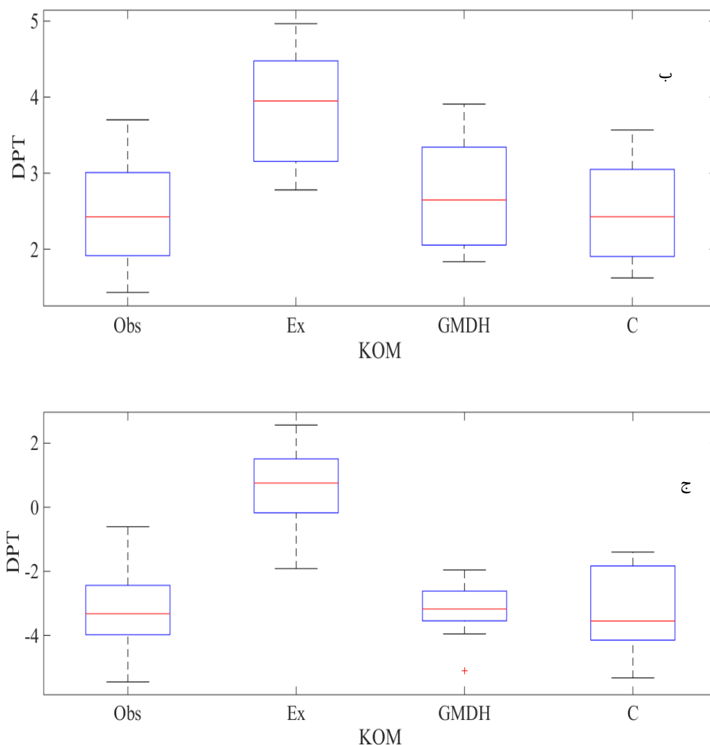
شکل ۵: نمودار مقادیر دمای نقطه شبنم؛ مشاهداتی (Obs) و پیش‌بینی با روش رگرسیون حداقل مربعات (C).
