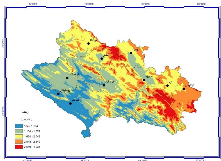
شکل (۱) نقشه توزیع جغرافیایی ایستگاه های مورد مطالعه
