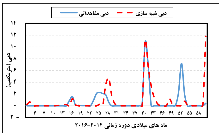
شکل ۵: مقایسه هیدروگراف‌های شبیه‌سازی شده و مشاهداتی در دوره اعتبارسنجی ایستگاه خنداب
