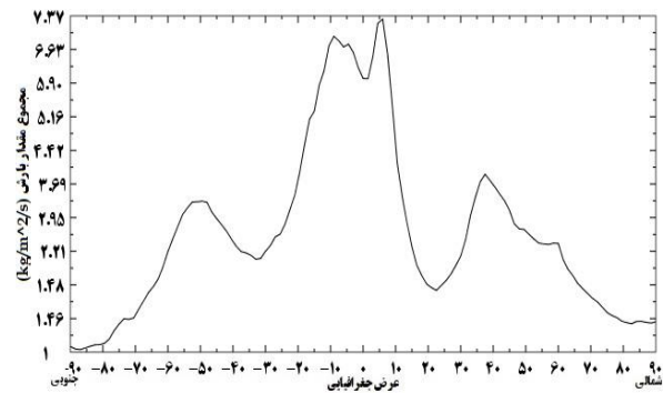
شکل ۱۰: میانگین زمانی ساختار افقی بارش ( \text{kg/m}^2/\text{s} ) از سال ۱۹۷۹-۲۰۱۸
