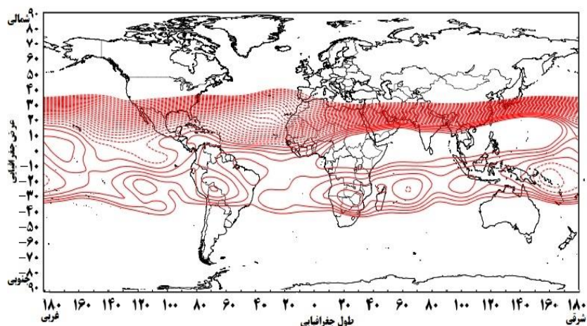
شکل ۱۳: میانگین زمانی ساختار افقی سلول هادلی ( 10\text{kg/s} ) در هر دو نیمکره در سطح ۱۰۰۰ تا ۱۰۰ هکتوپاسکال از سال ۱۹۷۹-۲۰۱۸
