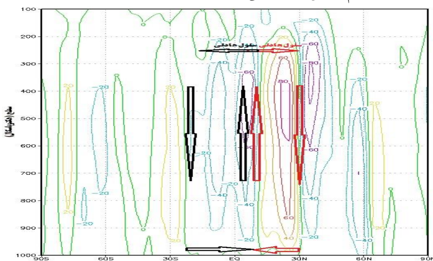
شکل ۱۲: میانگین زمانی ساختار عمودی سلول هادلی ( 10\text{kg/s} ) در سطح ۱۰۰۰ تا ۱۰۰ از سال ۱۹۷۹-۲۰۱۸
