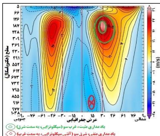
شکل ۲: ساختار قائم میانگین زمانی باد مداری (m/s) از سطح ۱۰۰۰ تا سطح ۵ هکتوپاسکال از سال ۲۰۱۸-۱۹۷۹
