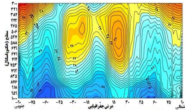
شکل ۹: میانگین زمانی ساختار عمودی رطوبت نسبی (%) در سطح ۱۰۰۰ تا ۳۰۰ هکتوپاسکال از سال ۱۹۷۹-۲۰۱۸
