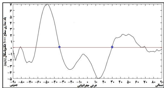
شکل ۴: لبه عرض جغرافیایی سلول هادلی با باد مداری سطح صفر در سطح ۱۰۰۰ هکتوپاسکال (m/s) از سال ۱۹۷۹-۲۰۱۸
