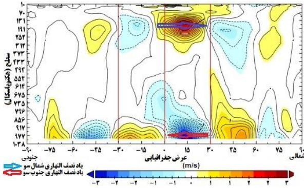
شکل ۶: ساختار عمودی میانگین زمانی باد نصف‌النهاری (m/s) در سطح ۱۰۰۰ تا ۱۰۲۸ هکتوپاسکال از سال ۱۹۷۹-۲۰۱۸
