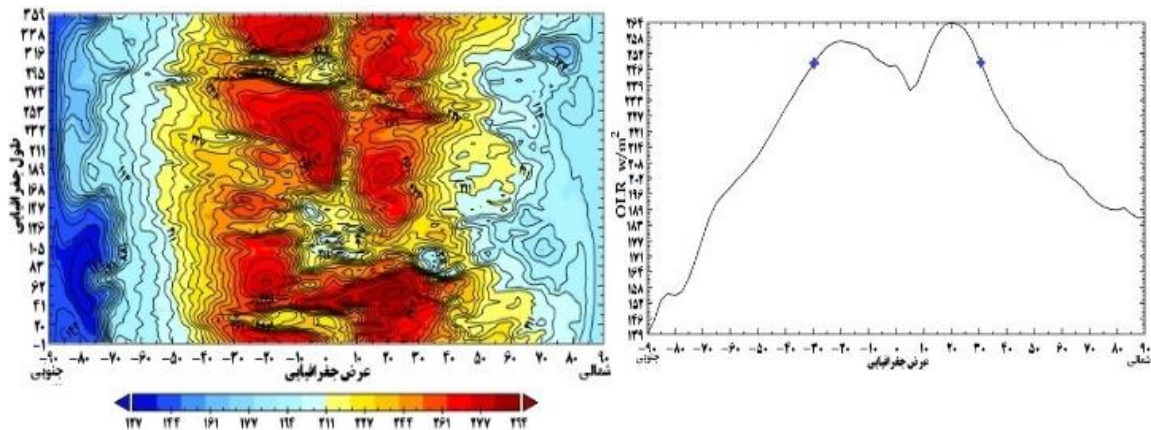
شکل ۱۱: میانگین زمانی ساختار عمودی تابش موج بلند خروجی زمین ( \text{W/m}^2 ) از سال ۱۹۷۹-۲۰۱۸
