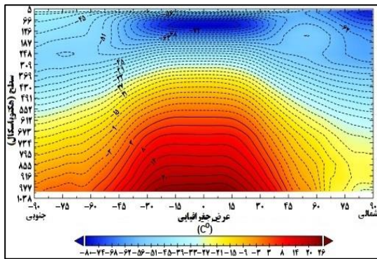
شکل ۱: میانگین زمانی ساختار عمودی دمای هوا (C) در سطح ۵ تا ۱۰۰۰ هکتوپاسکال از سال ۲۰۱۸-۱۹۷۹
