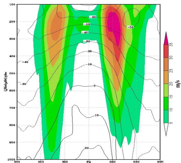
شکل ۵: نقشه ترکیبی میانگین زمانی دمای هوا (خطوط سیاه، C) و باد مداری (رنگ‌های سایه دار، m/s) از سال ۱۹۷۹-۲۰۱۸
