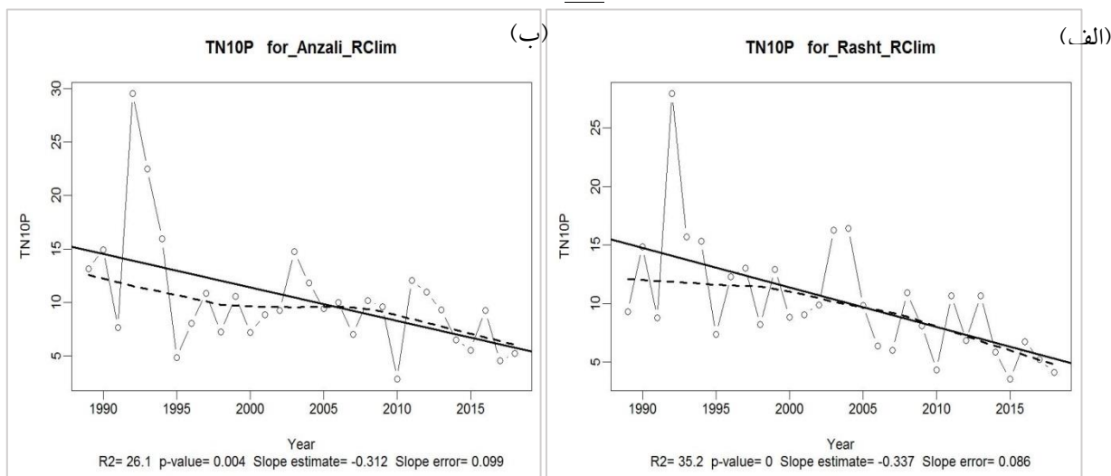
شکل ۷- نمودار نمایه شب‌های سرد (TN10p) با نرم افزار (RClindex) در دوره بلند مدت منتهی به ۲۰۱۸، (الف) رشت، (ب) انزلی
