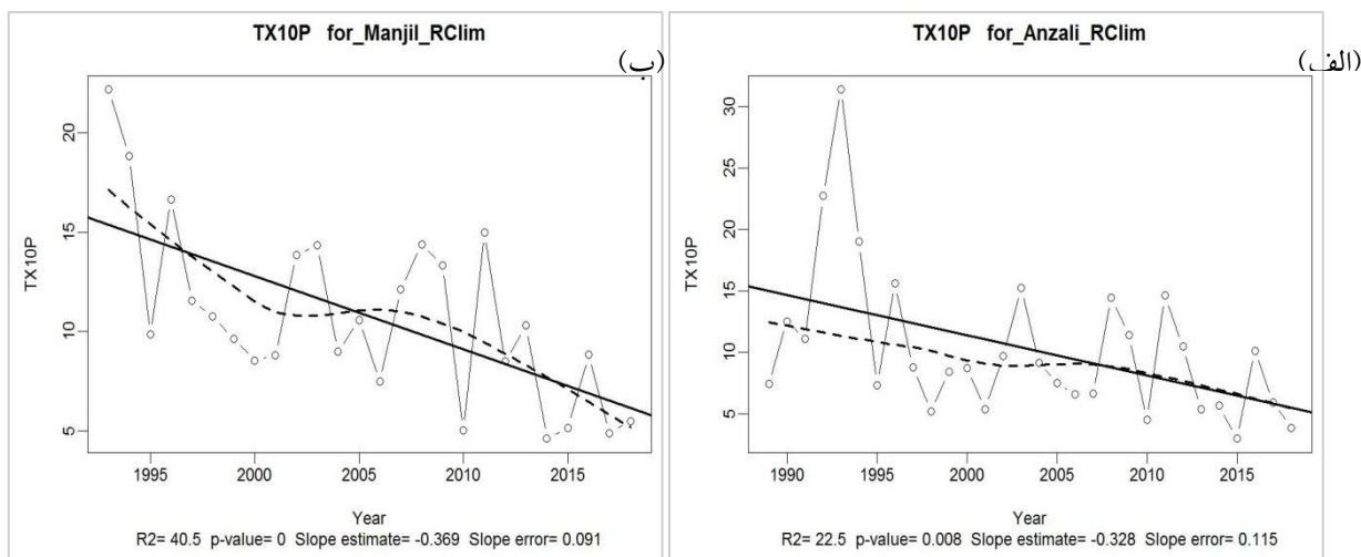
شکل ۶- نمودار نمایه روزهای سرد (TX10p) با نرم افزار (RClindex) در دوره بلند مدت منتهی به ۲۰۱۸، (الف) انزلی، (ب) منجیل
