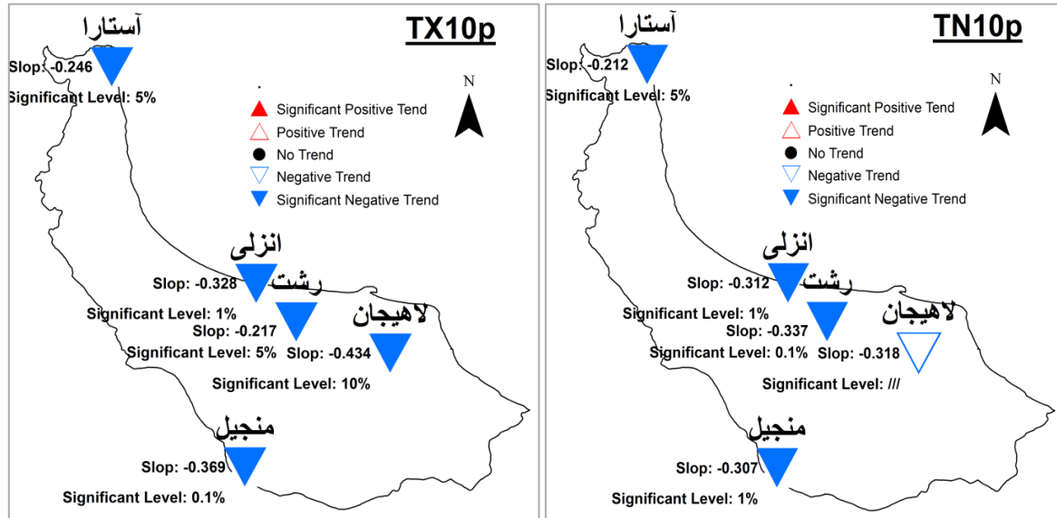
شکل ۸- روند دو نمایه دمایی سرد برای پنج شهرستان گیلان، (الف) تعداد روزهای تابستانی (TX10p) و (ب) تعداد شب های حاره ای (TN10p)، در دوره بلند مدت منتهی به ۲۰۱۸
