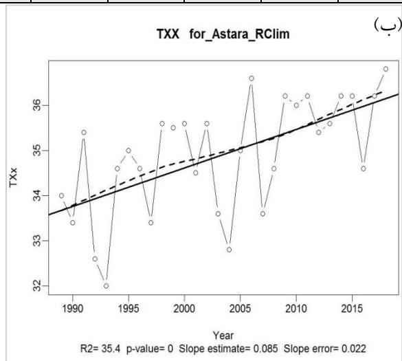
شکل ۳- نمودار نمایه بیشینه دمایی روزانه (TXx) با نرم افزار (RCLimdex) در دوره بلند مدت منتهی به ۲۰۱۸، (الف) رشت، (ب) آستارا
