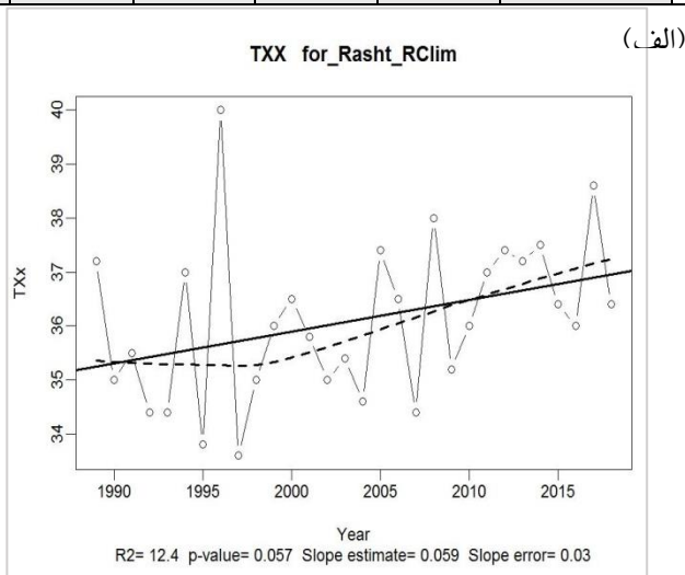
شکل ۳- نمودار نمایه بیشینه دمایی روزانه (TXx) با نرم افزار (RCLimdex) در دوره بلند مدت منتهی به ۲۰۱۸، (الف) رشت، (ب) آستارا
