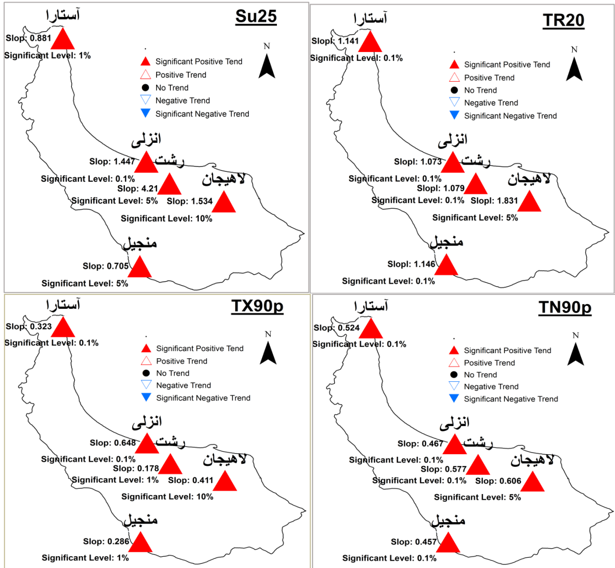
شکل ۵- روند تعدادی نمایه‌های دمایی گرم برای پنج شهرستان گیلان، (الف) تعداد روزهای تابستانی (Su25)، (ب) تعداد شب‌های حاره‌ای (TR20)، (ج) روزهای گرم (TX90p) و (د) شب‌های گرم (TN90p) در دوره بلند مدت منتهی به ۲۰۱۸
