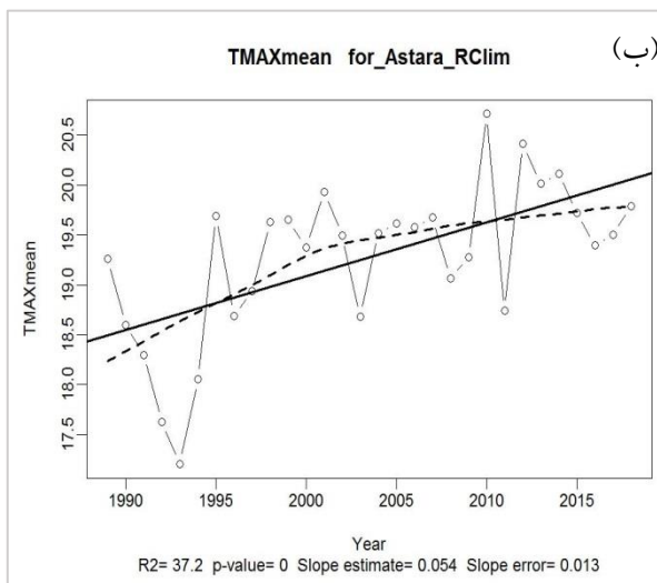
شکل ۹- میانگین دمای بیشینه (TMAXmean) با نرم افزار (RCLIMDEX) در دوره بلند مدت منتهی به ۲۰۱۸، (الف) انزلی، (ب) آستارا
