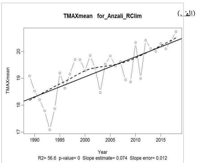
شکل ۹- میانگین دمای بیشینه (TMAXmean) با نرم افزار (RCLIMDEX) در دوره بلند مدت منتهی به ۲۰۱۸، (الف) انزلی، (ب) آستارا
