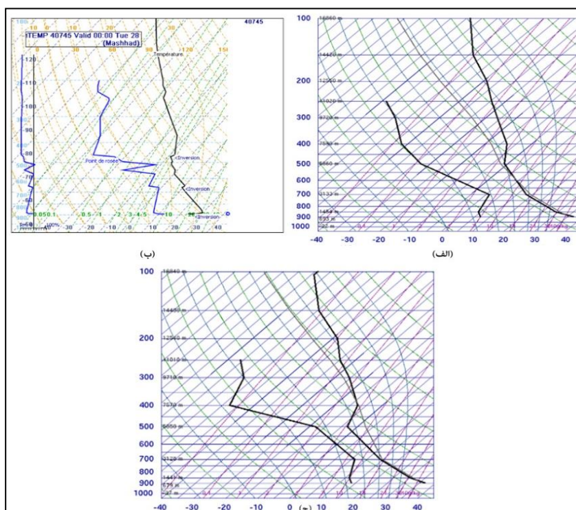
شکل ۴. نمودارهای ترمودینامیکی (اسکیوتی) جو بالای مشهد در روز (الف) ۲۷ جولای ۲۰۰۹ ساعت ۱۲ (UTC)، (ب) ۲۸ جولای ۲۰۰۹ ساعت ۰۰ و (ج) ۲۸ جولای ۲۰۰۹ ساعت ۱۲ (UTC)
