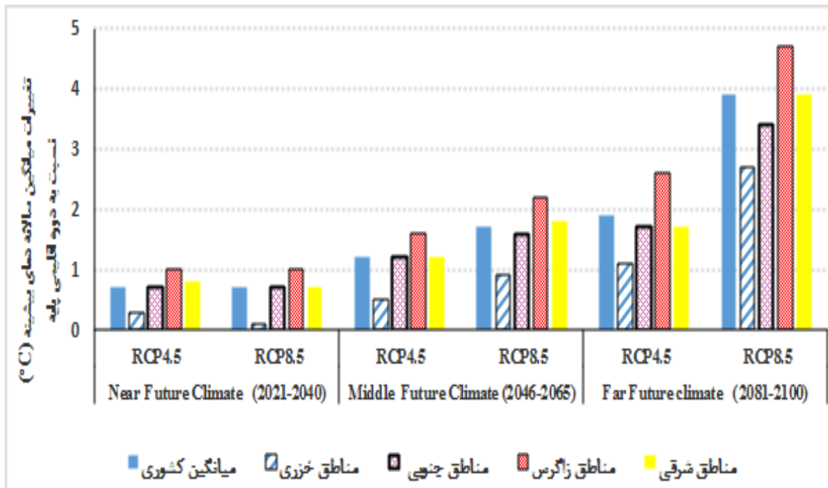
شکل ۵- تغییرات میانگین سالانه دمای بیشینه (°C) منطقه‌ای (میانگین کشوری) و میانگین ناحیه‌ای ایران نسبت به میانگین دوره اقلیمی پایه (۱۹۸۶-۲۰۰۵)، در چشم انداز آتی (اقلیم آتی نزدیک، میانی و دور) تحت سناریوهای مختلف RCP-نگرش یکپارچه
