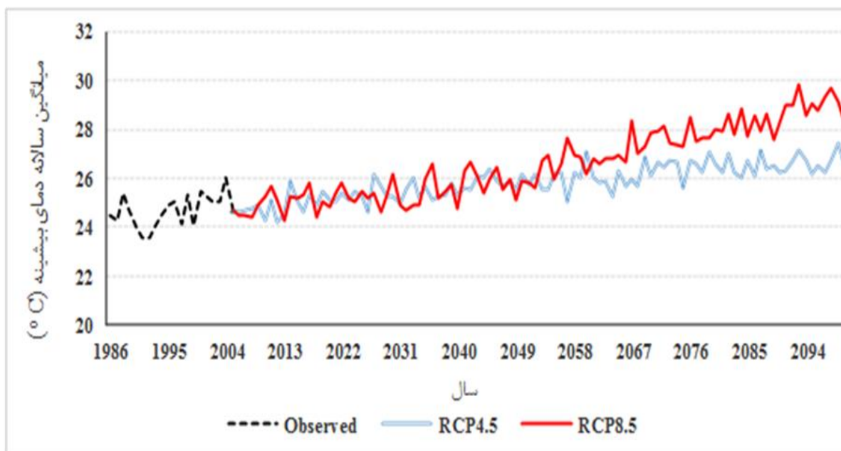
شکل ۶- سری زمانی میانگین سالانه دمای بیشینه ایران در اقلیم پایه و آتی تحت سناریوهای RCP
