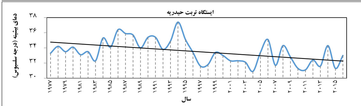
شکل ۲- روند تغییرات دمای بیشینه در ایستگاه‌های با بیش‌ترین شیب روند ماهانه
