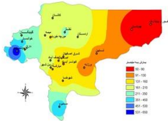
شکل ۱۲- پهنه‌بندی استان اصفهان بر اساس بارش سال زراعی ۹۳-۱۳۹۲ خورشیدی (از هواشناسی استان اصفهان)
