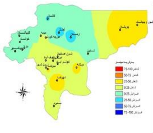
شکل ۱۳- درصد افزایش یا کاهش بارش سال زراعی ۹۳-۱۳۹۲ نسبت به سال گذشته (از هواشناسی استان اصفهان)
