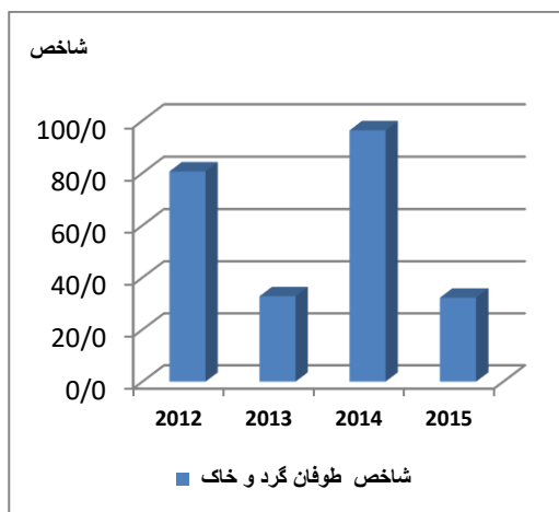
شکل ۱۰- میانگین سالانه شاخص طوفان گرد و خاک استان اصفهان در دوره آماری
