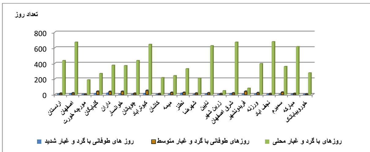
شکل ۷- میانگین شاخص DSI در نقاط مختلف استان اصفهان در طول دوره آماری ۲۰۱۵-۲۰۱۲ میلادی
