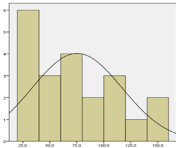
شکل ۵- بافت نگار داده‌های DSI و شرایط آنها نسبت به منحنی نرمال
