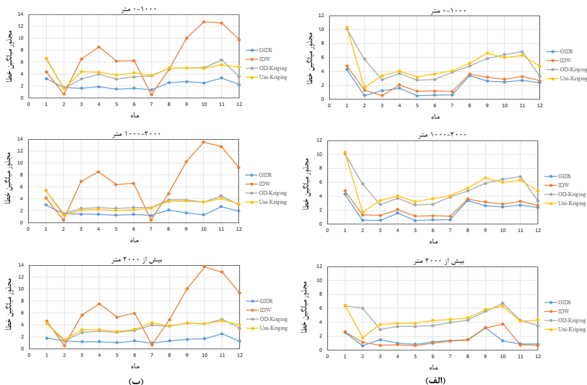
شکل ۴. مجذور میانگین خطای چهار روش برای (الف) دمای بیشینه (ب) دمای کمینه در بازه ارتفاعی ۰ تا ۱۰۰۰ متر، ۱۰۰۰ تا ۲۰۰۰ متر و بیش از ۲۰۰۰ متر از سطح دریا
