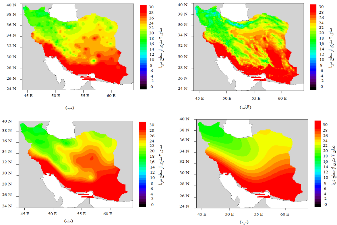
شکل ۶- الف. پهنه‌بندی میانگین دمای بیشینه سالانه مربوط به چهار روش (الف) GIDS، (ب) IDW، (پ) OD-Kriging و (ت) Uni-Kriging
