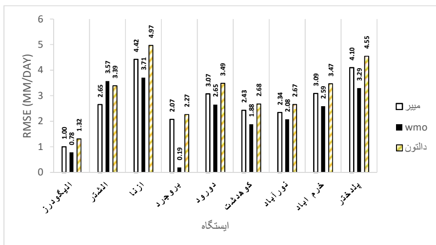
شکل ۱۱- مقادیر RMSE تخمین تبخیر تعرق مرجع با روش‌های مبتنی بر انتقال جرم در ایستگاه‌های مورد مطالعه
