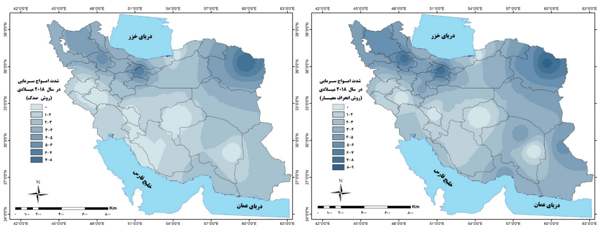
شکل ۷- شدت امواج سرمای در سال ۲۰۱۸ میلادی برحسب درجه سانتیگراد (بالا: روش انحراف معیار، پایین: روش صدک)
