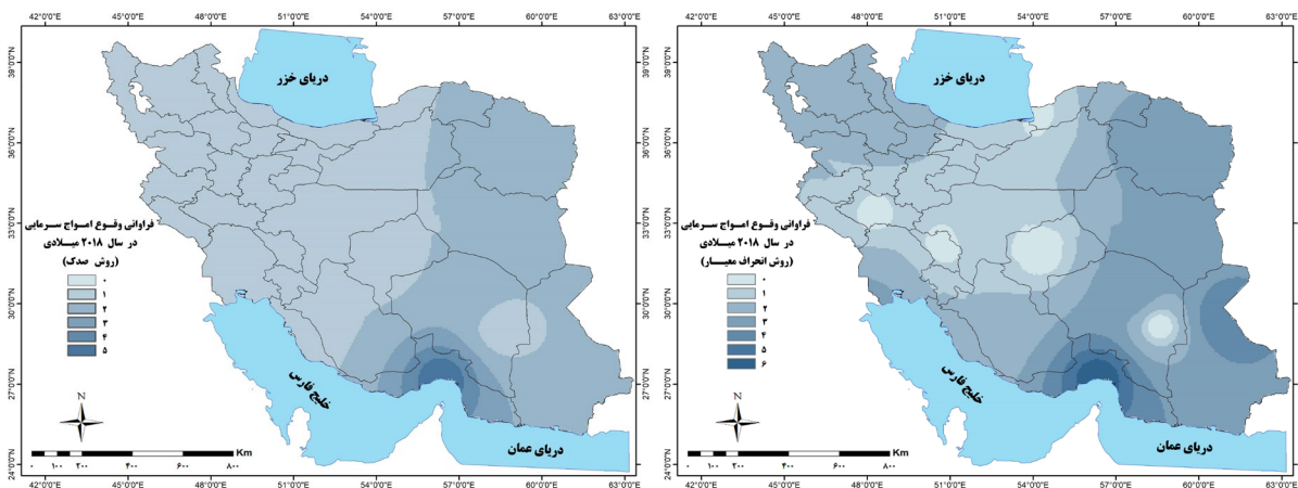
شکل ۶- فراوانی وقوع امواج سرمای کشور در سال ۲۰۱۸ میلادی (بالا: روش انحراف معیار، پایین: روش صدک)
